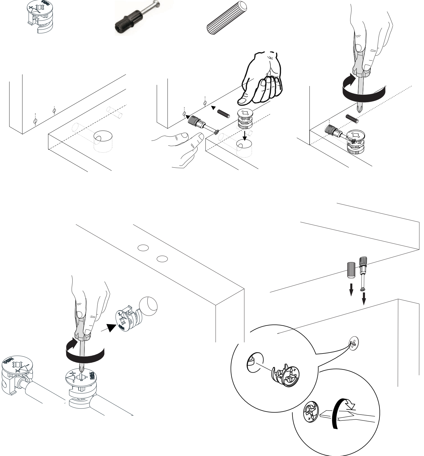
Minifix Gövde
