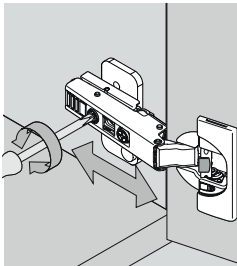
Tiefenverstellung
