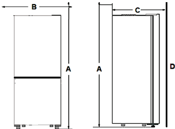
RAUMBEDARF DES GERÄTES INKL. DER MINDESTABSTÄNDE FÜR EINE ORDNUNGSGEMÄßE BELÜFTUNG BEI GESCHLOSSENEN TÜREN
