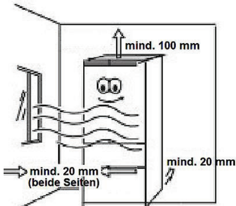
RAUMBEDARF DES GERÄTES INKL. DER MINDESTABSTÄNDE FÜR EINE ORDNUNGSGEMÄßE BELÜFTUNG BEI GESCHLOSSENEN TÜREN
