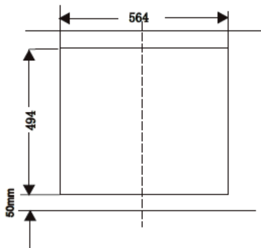
Abbildung 3 Ausschnitt Arbeitsplatte
