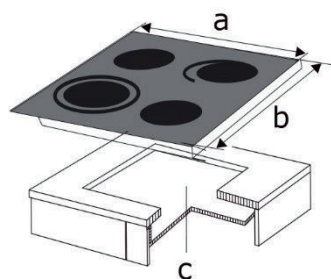
Abbildung 4 Glaskeramikkochfeld
